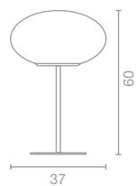
ART. 2466 Lampada da tavolo /Table lamp Ø 37 h 60 cm 1 x E27
