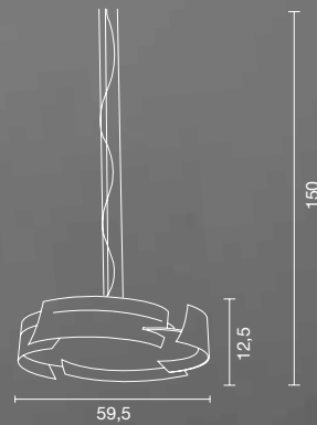
ART. 1024E Sospensione /Suspension Ø 59,5 h 12,5 h max 150 cm 4 x E27
