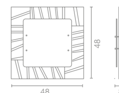
ART. 0651 Plafoniera /Ceiling lamp 48 x 48 h 8 cm 4 x E27
