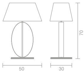
ART. 1085 Lampada da tavolo /Table lamp 50 x 30 h 70 cm 1 x E27 Kg. 5,7 CE IP 20
