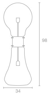
ART. 2751 Lampada da appoggio / Floor lamp Ø 34 h 98 cm 2 x E27
