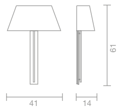
ART. 1084 Applique /Wall lamp 41 h 61 P.14 2 x E14 Kg. 1,2 CE IP 20
