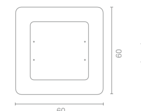
ART. 0612 Plafoniera /Ceiling lamp 60 x 60 h 8 cm 4 x E27
